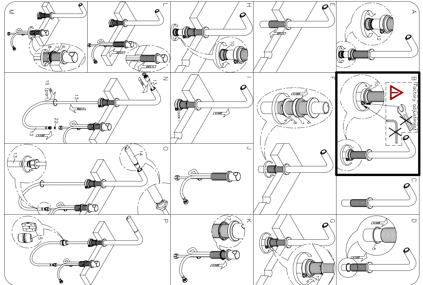
HI-144P (B)
